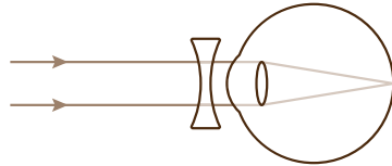
Bijziend oog met min-glas
