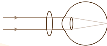
Verziend oog met plus-glas
